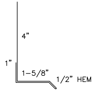
DRIP EDGE (DF022)
